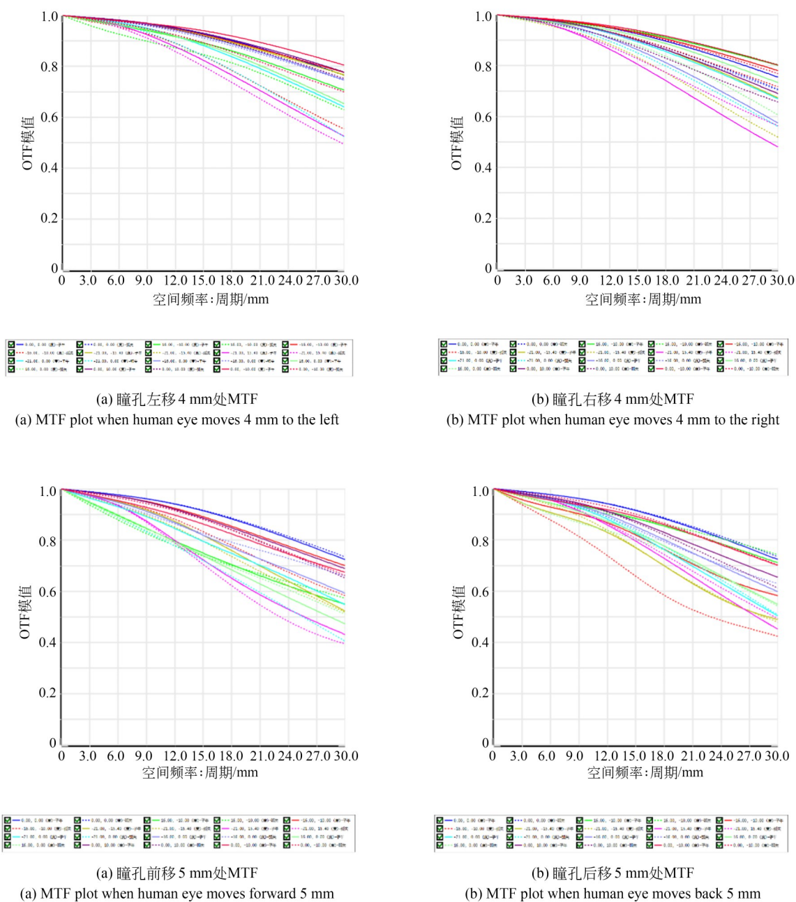
图7 瞳孔偏移至4个不同位置时光学系统的MTF
